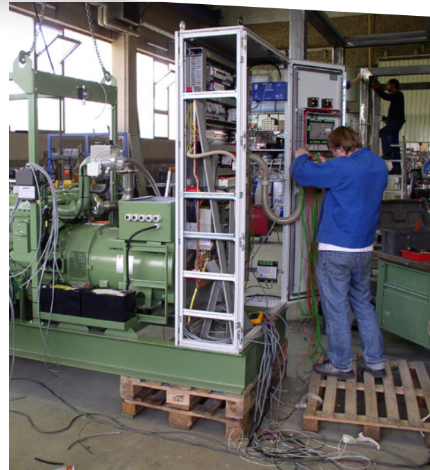
Aufbau und Verkabelung einer Gasgeneratoranlage Construction and processing of a gas generator
