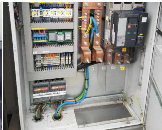
Direktanschluss auf Schiene: Max. 240 2 - M12 Kabelschuh
